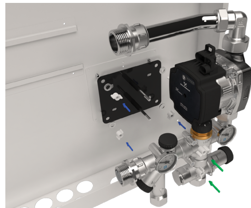
Sekoitusryhmän konsoli VS2:n asennus.
