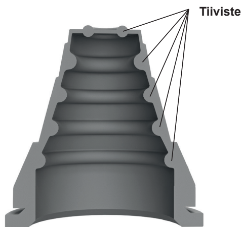
Putkiläpiviennin läpileikkauksesta näet tiivisteiden sijainnin.
