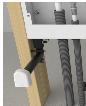
Viemäröintikulma liitettynä suoraan kaapin ylivuotoputken kaulukseen päätyy samaan tilaan kuin kaapin huoltoaukko tai vaihtoehtoisesti sen takana olevaan tilaan.
