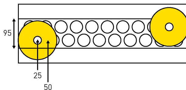
Esimerkki: asennus, jossa on syöttöputken eristys. Kuvassa olevan kaapin syvyys on 95 mm.
