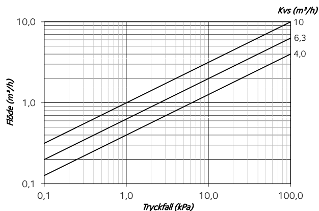
KAPACITETSDIAGRAM
