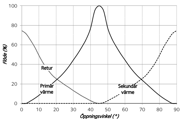
VENTILKARAKTÄRISTIK
