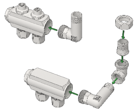
Liitäntäyhteen asennus 2-lähtöiseen LK Minijakotukkiin.
