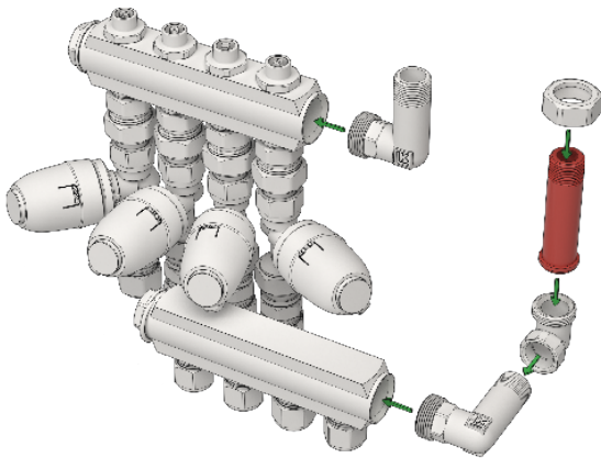
Liitäntäyhteen asennus 4-lähtöiseen LK Minijakotukkiin ja jatkoputkella (näkyv. punaisena) varustettuun LK Termostaattiventtiilisarjaan Mini.
