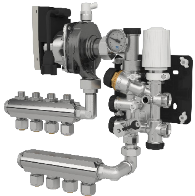
LK Minijakotukki kytkettynä LK Minisekoitusryhmään M60n.
