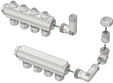
Liitäntäyhteen asennus 4-lähtöiseen LK Minijakotukkiin.
