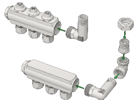
Liitäntäyhteen asennus 3-lähtöiseen LK Minijakotukkiin.
