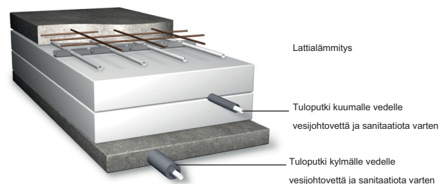
Suojaputkellisten putkien asennus betonilaattaan, jossa on lattialämmitys.
