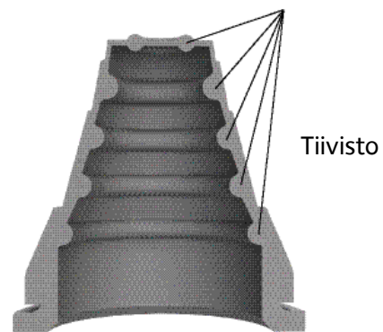
Putken läpiviennin LP 20-25 poikkileikkaus LK näyttää putken tiivisteen sijainnin.
