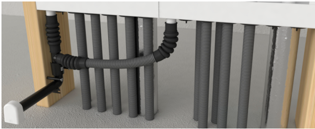
Ylivuotoputkien yhteenliittäminen.
