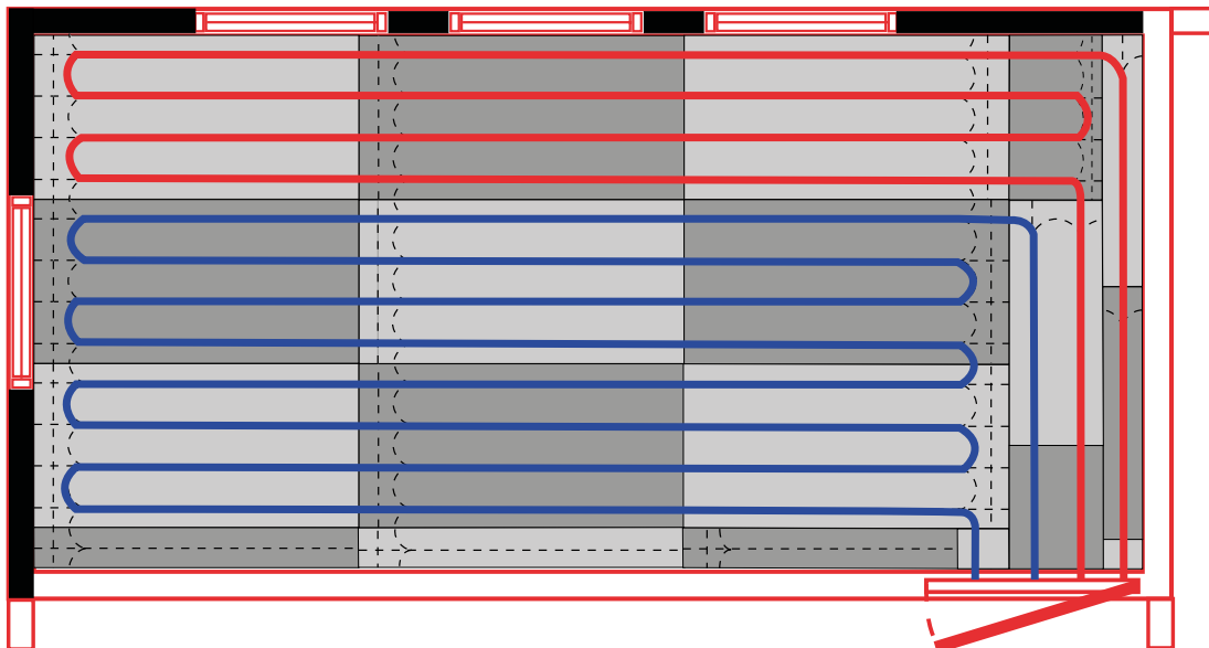
Esimerkkikuva. Kuvassa koeasettelu ja putkipiirit.
