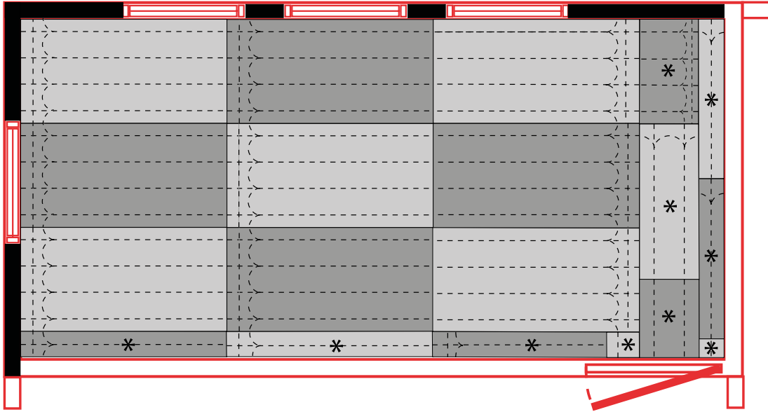
Esimerkkikuva. Kuvassa esimerkki levyjen koeasettelusta. * Katkaistut LK CombiBoard EPS -levyt.
